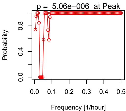
(d) Peak Significance
